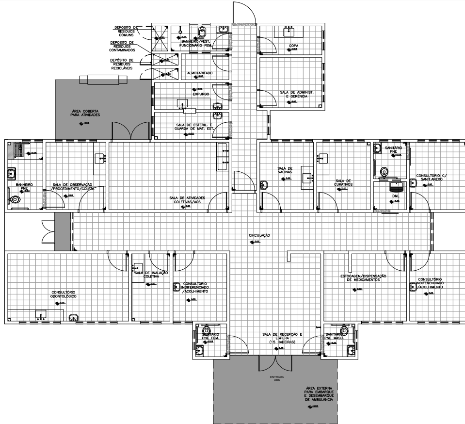
Planta Baixa Acabamento Piso
