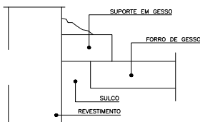
Detalhe -Junta de Dilatação Sem Escala
