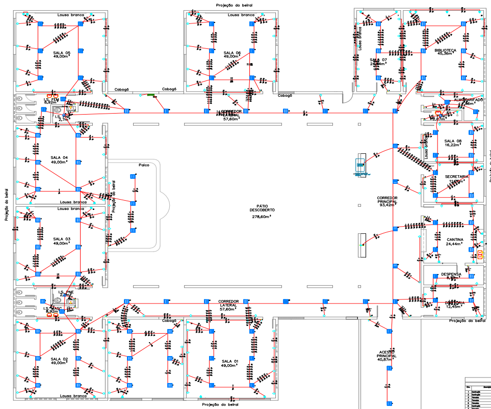
2 PLANTA - PROPOSTA 1 ESCALA 1 : 100
