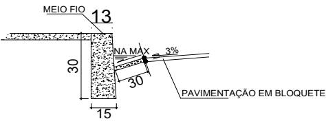
DETALHE "A" - SARJETA ESC: 1/10
