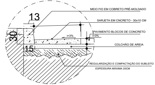
DETALHE 01 - MEIO-FIO E SARJETA - PISO BLOCO DE CONCRETO ESCALA: 1/25
