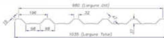
Figura 2 – imagem telha metálica trapezoidal TP40-980
