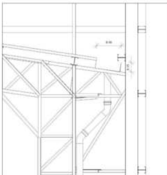
Figura 2 - Imagem das calhas
