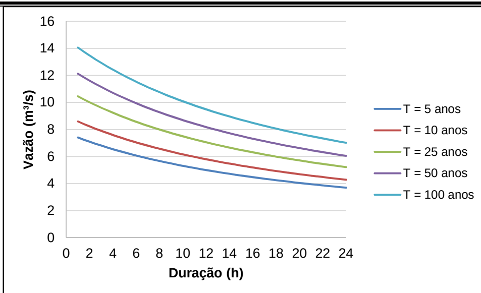
Figura 6.126 – Vazões estimadas pelo método racional para a MB 03 com período de retorno de 5 a 100 anos e intensidade de 1 a 24 horas.
