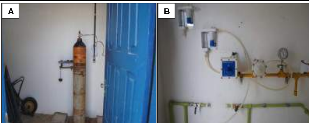
Figura 6.65 – Sistema de dosagem de cloro. Fonte: DRZ Geotecnologia e Consultoria (2015).
