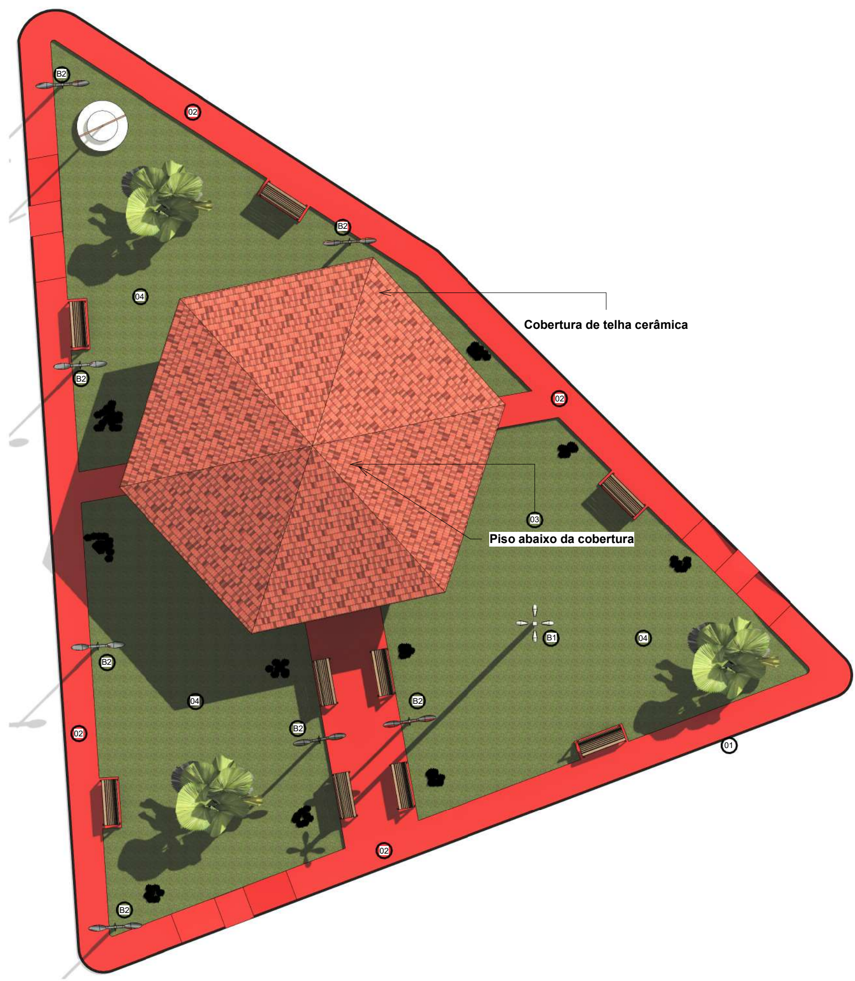
1 Planta de Layout 1 : 150
